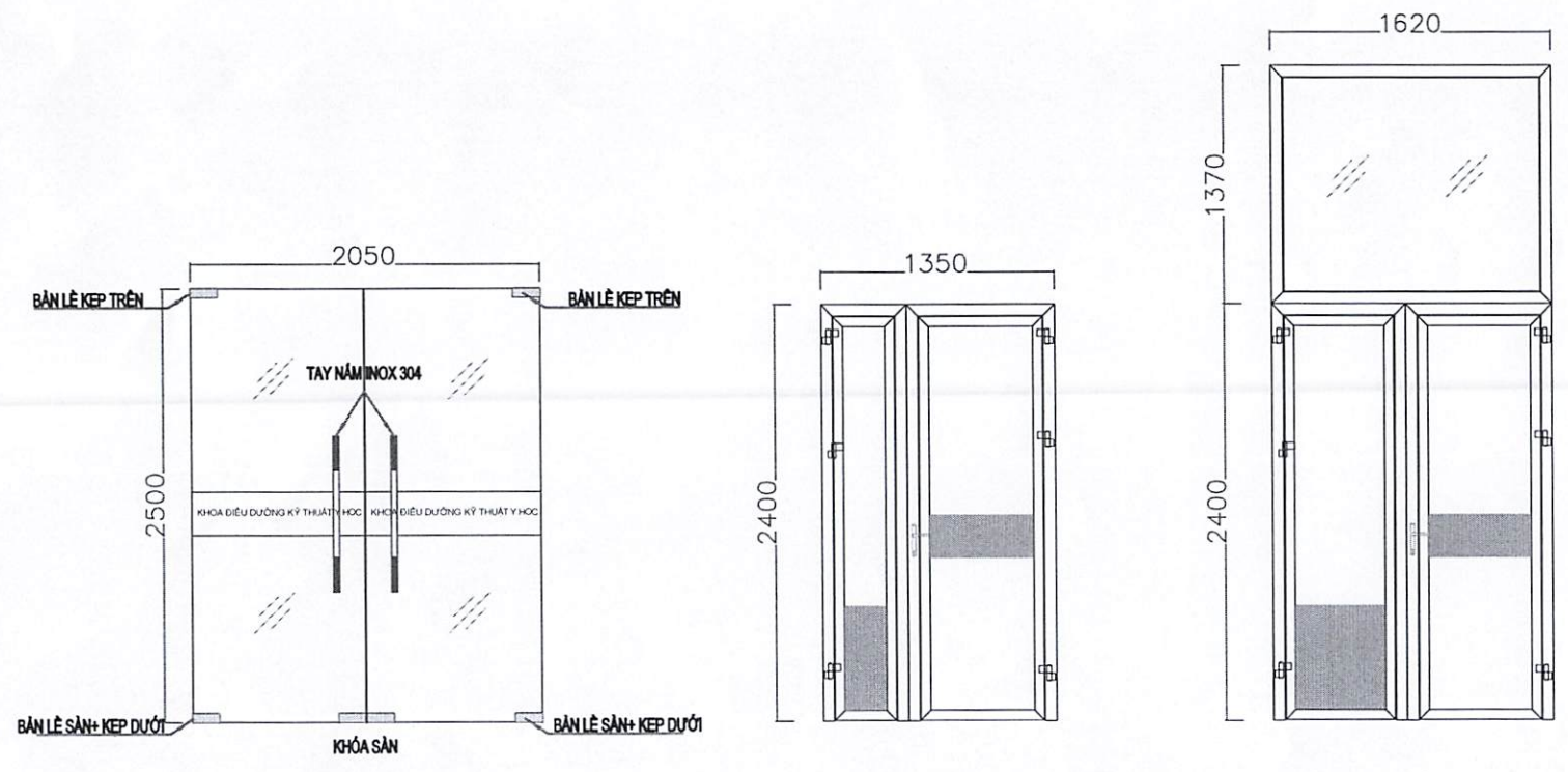
BẢN VẼ CHI TIẾT CỬA KHOA DƯỢC TL 1/40
